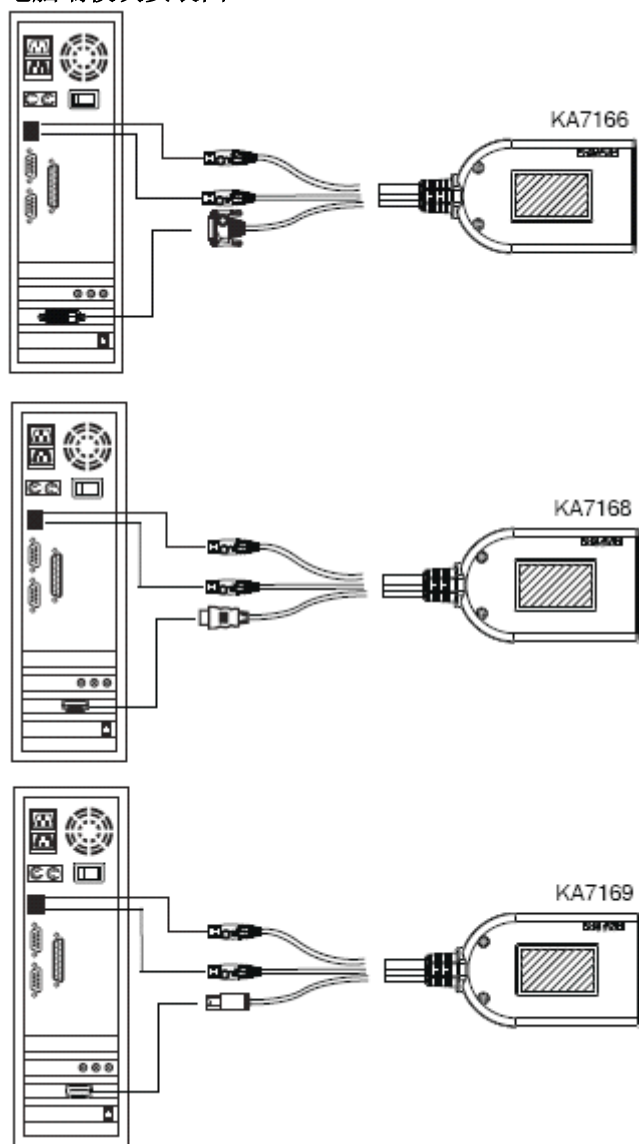
电脑端模块安装图-2
