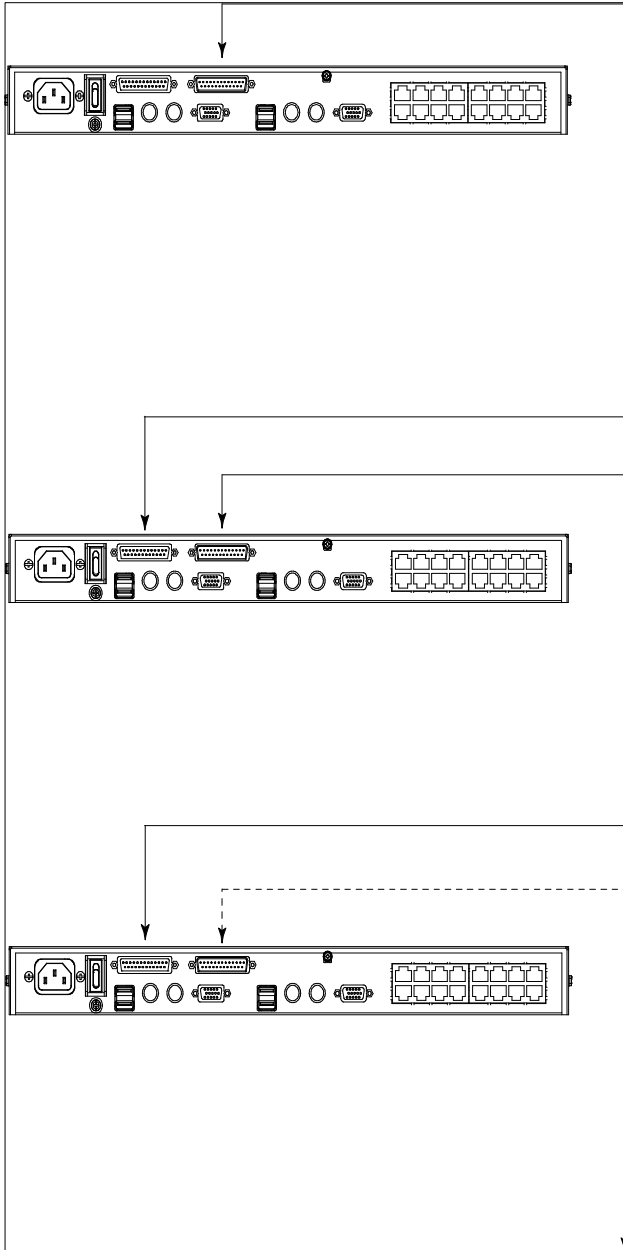
菊式串联安装图
